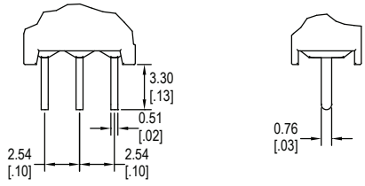
C SPDT
